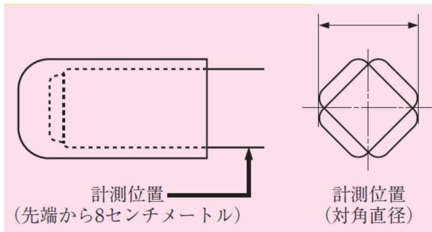
ちくとうの最小直径値の計測方法
